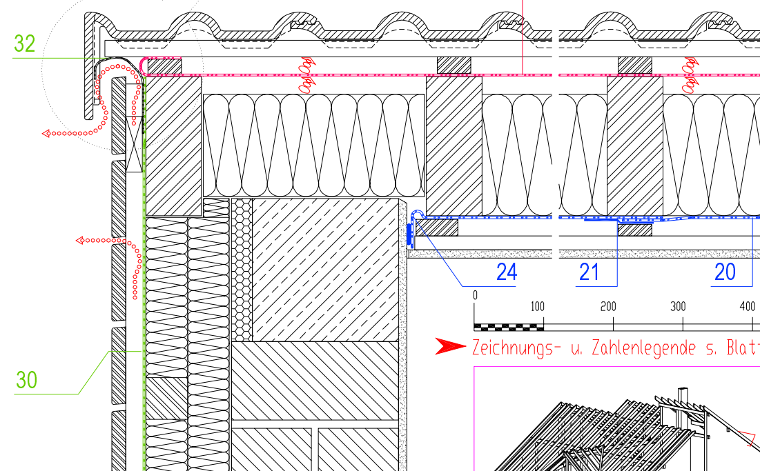
Offene hinterlüftete Wandverkleidung
