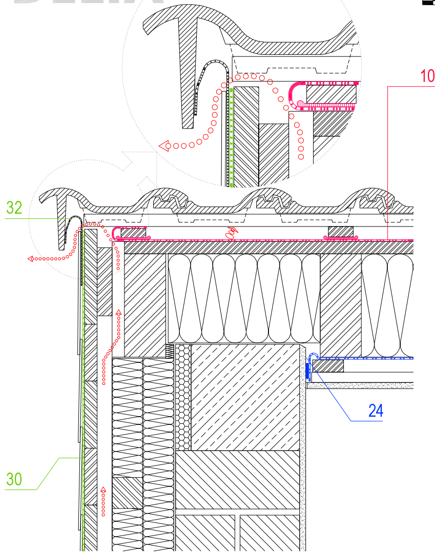
Geschlossene hinterlüftete Wandverkleidung
