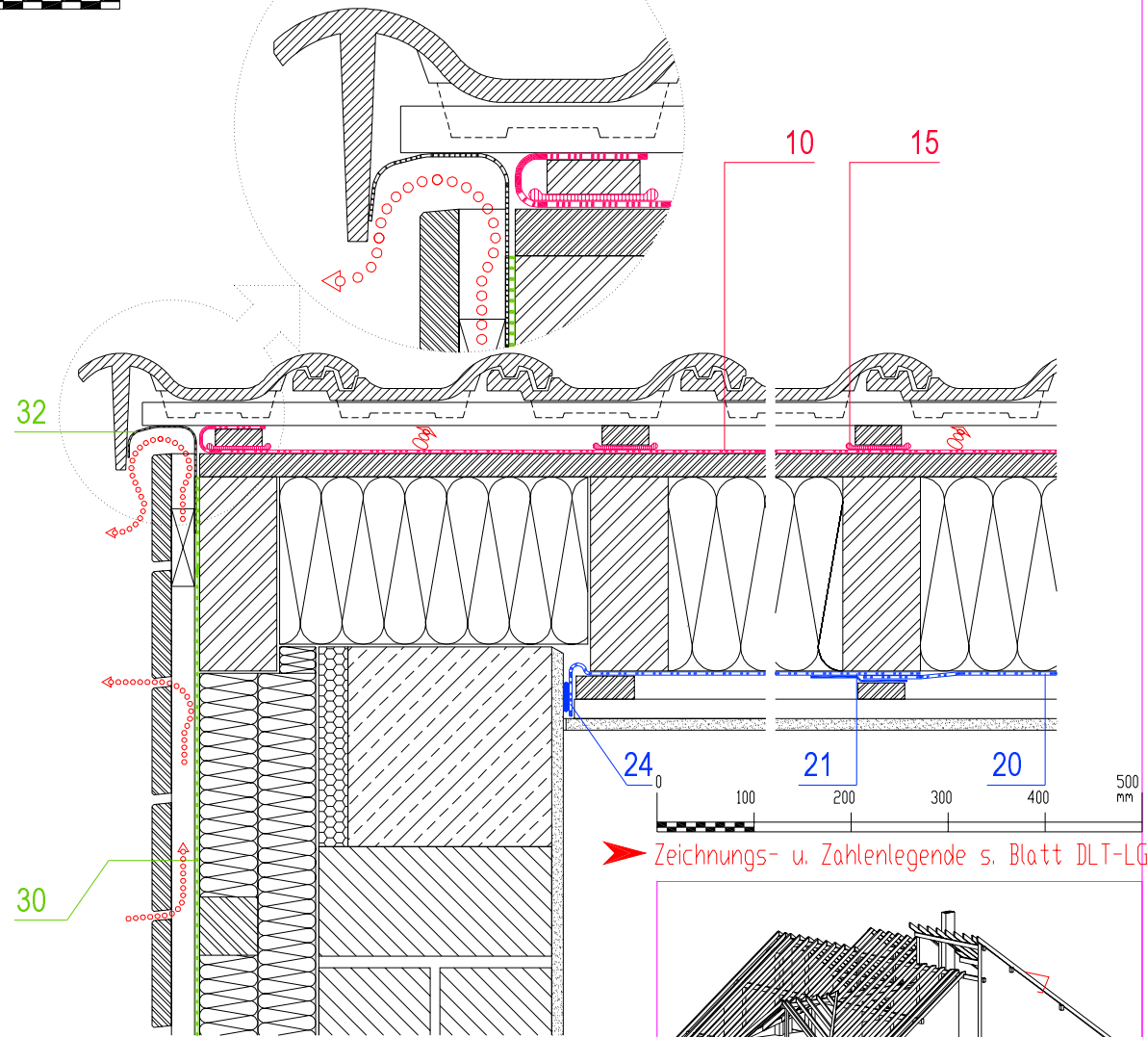
Offene hinterlüftete Wandverkleidung
