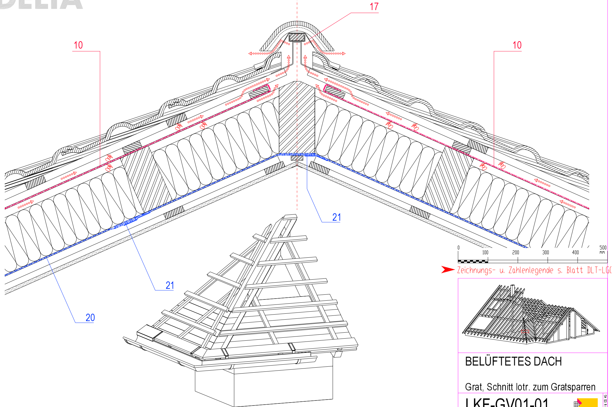
TEILISOMETRIE DACHKONSTRUKTION
