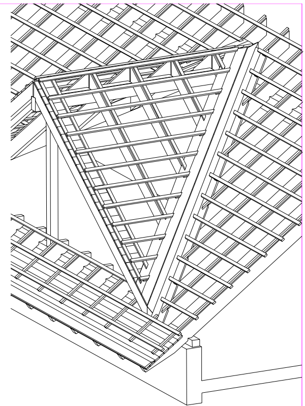
TEILISOMETRIE DACHKONSTRUKTION
