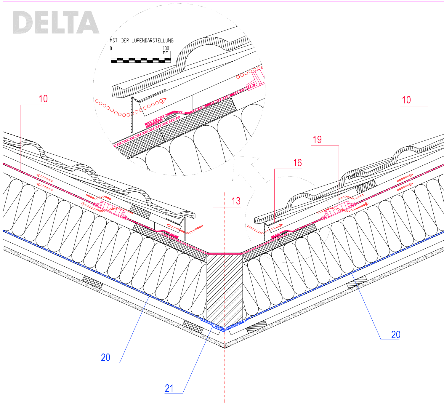
TEILISOMETRIE DACHKONSTRUKTION
