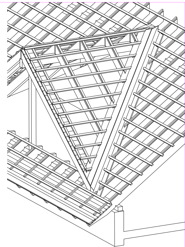
TEILISOMETRIE DACHKONSTRUKTION
