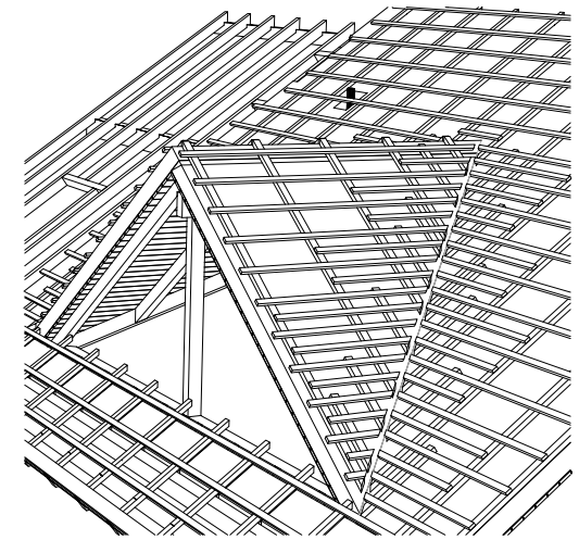
TEILPERSPEKTIVE (Kehlbereich)
