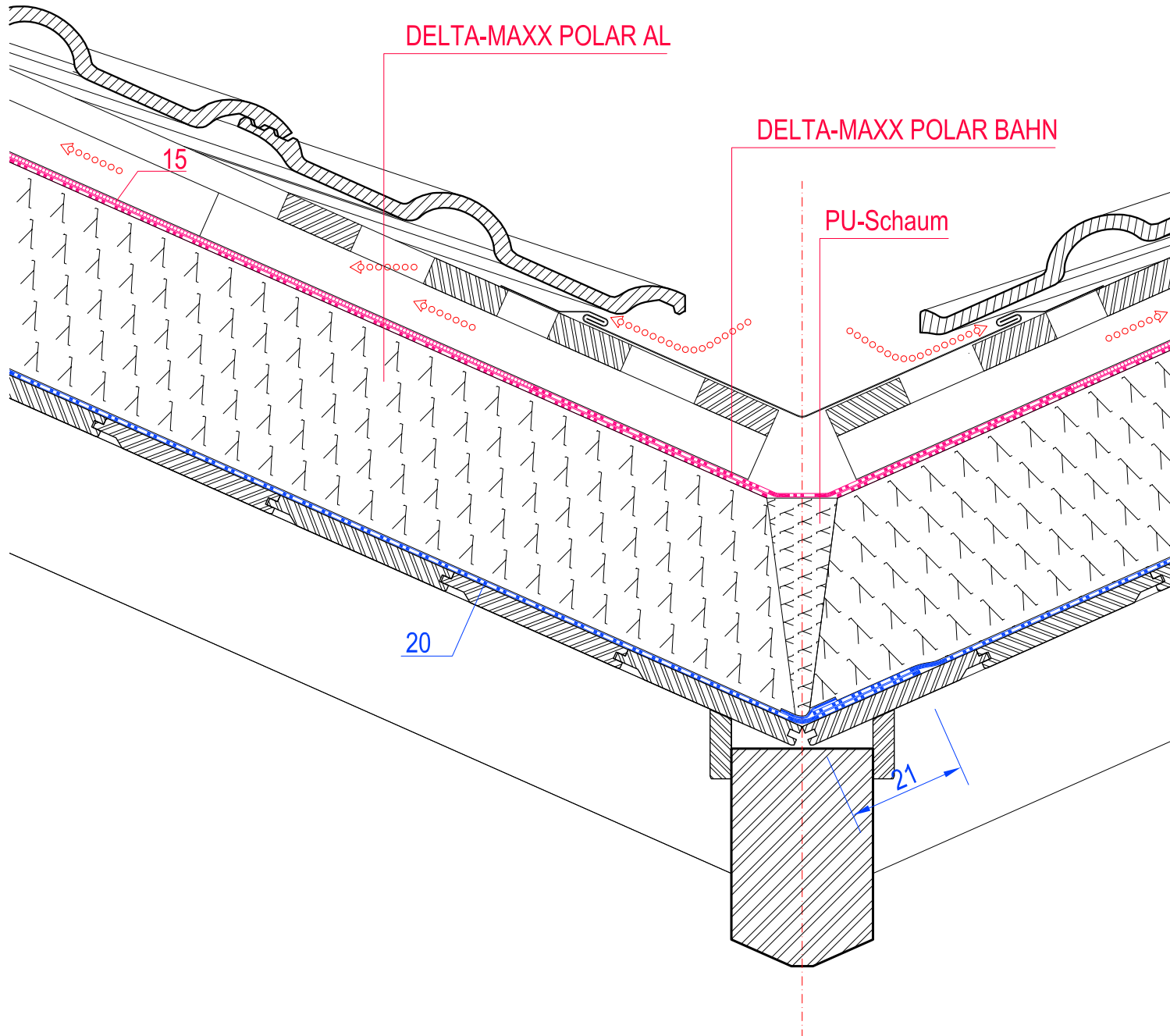
TEILPERSPEKTIVE (Kehlbereich)
