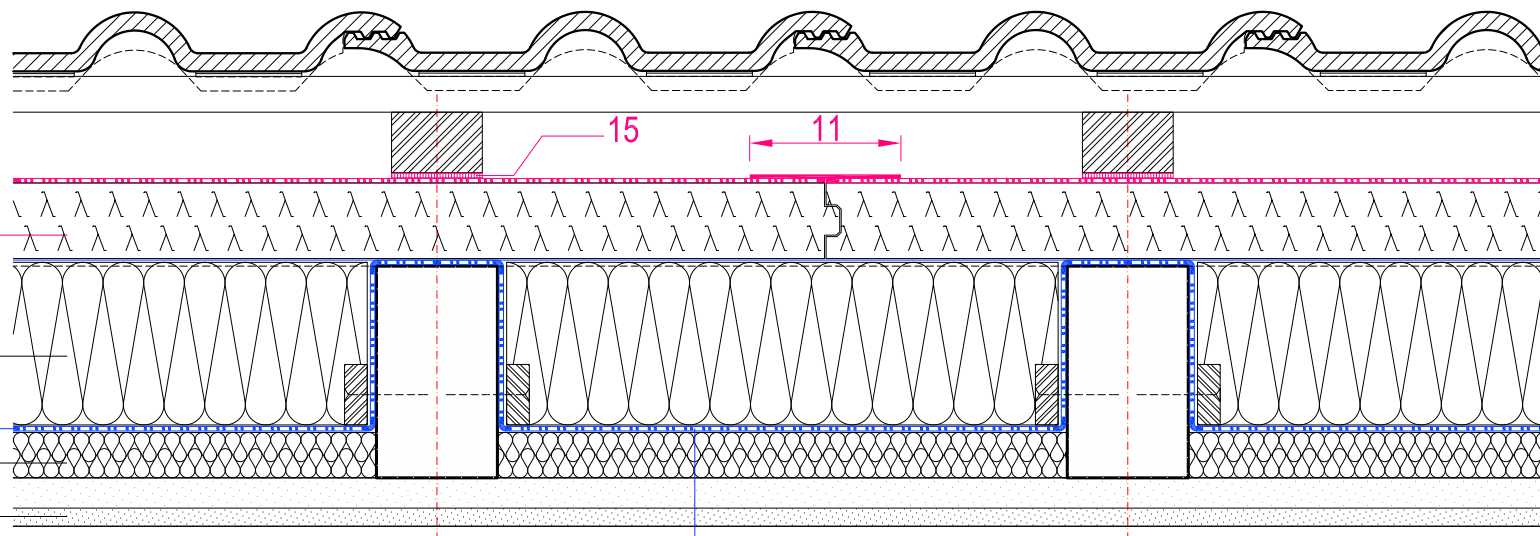
▲ REGELSCHNITT QUER
